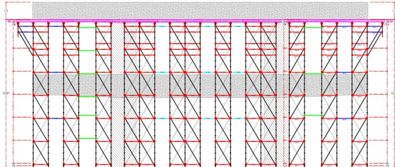
SECCIÓN LATERAL 5-5 DETALLE DE ALTURAS
